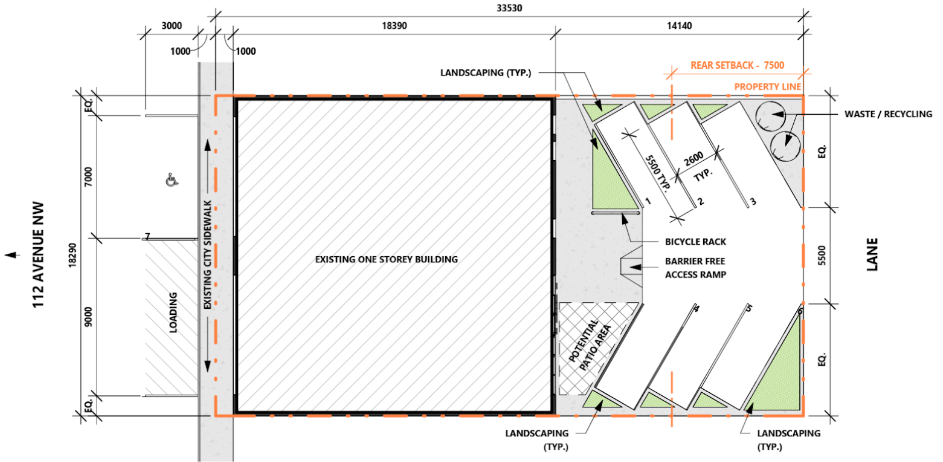
1 Site Plan A101 1 : 200
